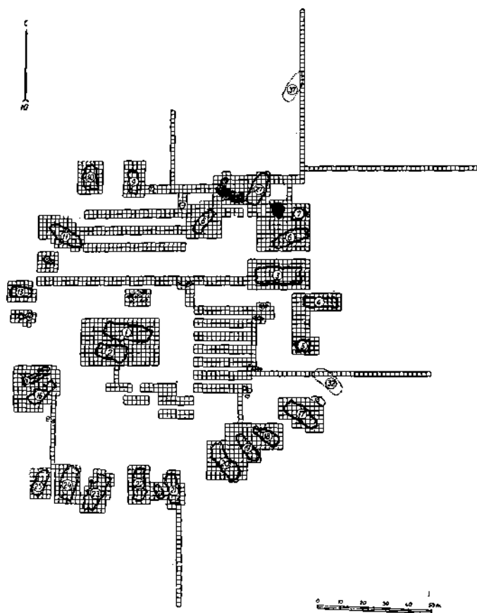
Рис. 1. Уроч. Коломийщина. Схематический план поселения (раскопки 1934—1938 гг.). Обозначения сплошной линией—раскопанные жилища, точками—«рянушечные кучи», пунктиром—нераскопанные еще жилища
